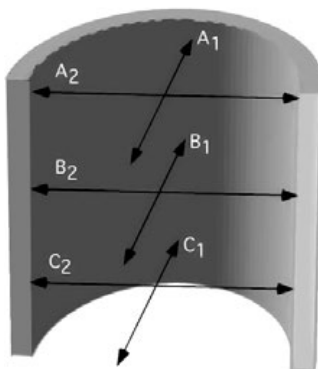
Medição do diâmetro interno do alojamento
